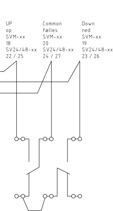
Opus 111763 (Jumper original pos.)
